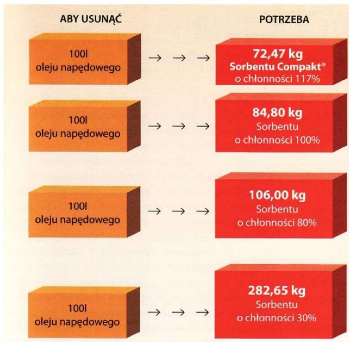
Rysunek nr 6.7. Przykładowe ilości potrzebnego sorbentu do różnych ropopochodnych 39
