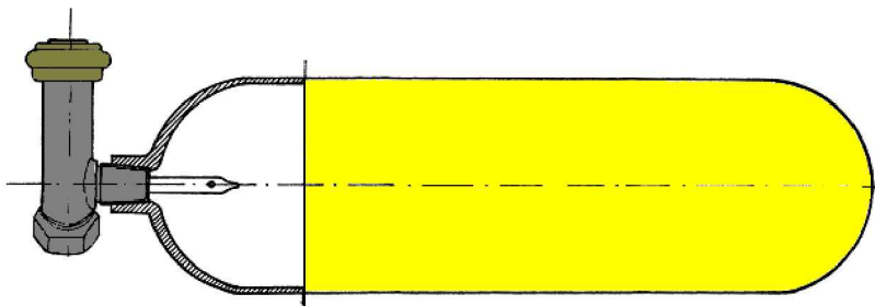
Rysunek nr 4.14. Butla stalowa na sprężone gazy
