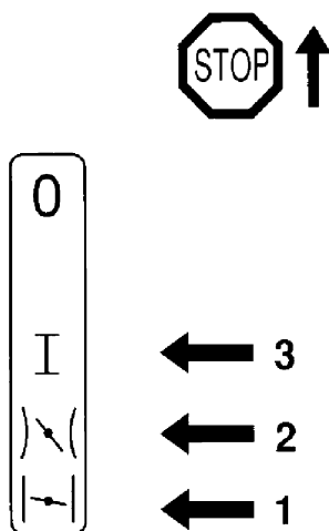
Rysunek nr 5.11. Przykładowe oznaczenia i położenia dźwigni sterowania gaźnikiem
