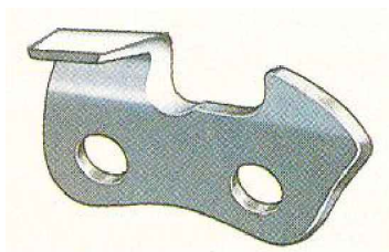
Rysunek nr 5.5. Ząb tnący stosowany w łańcuchach uniwersalnych przeznaczonych do ogólnego stosowania w leśnictwie, budownictwie, sadownictwie itp.
