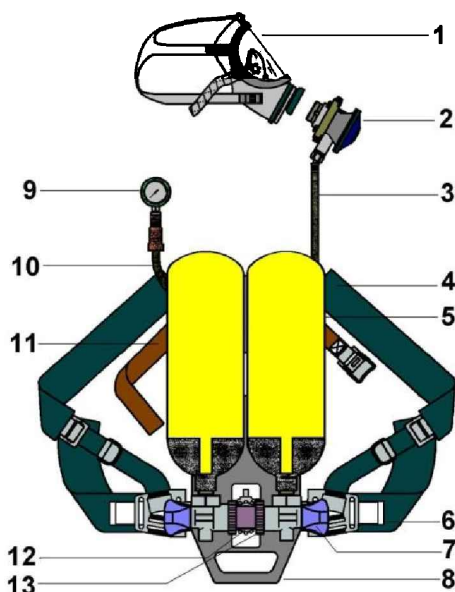
Rysunek nr 4.13. Części składowe aparatu powietrznego
