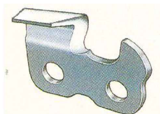
Rysunek nr 5.6. Ząb tnący stosowany w łańcuchach uniwersalnych przeznaczonych do malogabarytowych pil łańcuchowych.
