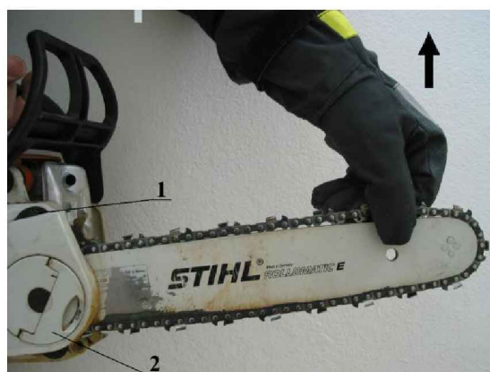
Fotografia nr 5.4. Prawidłowe napięcie łańcucha tnącego
