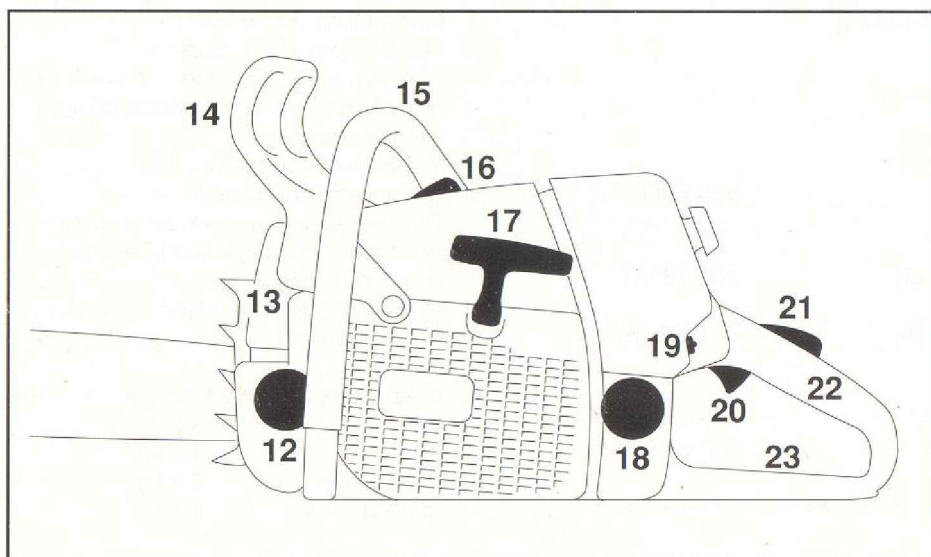
Rysunek nr 5.3. Podstawowe elementy pily łańcuchowej cd.:
